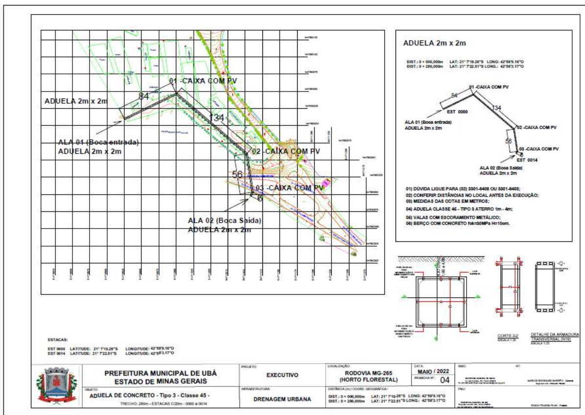
Figura 7 - Aduela de Concreto - Tipo 3 - Classe 45 - Trecho 280m
