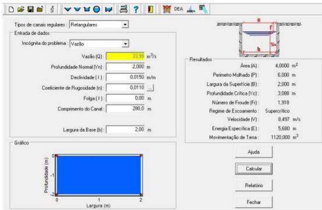
Figura 04 - SOFTWARE CANAL - GPRH/DEA-UFV
