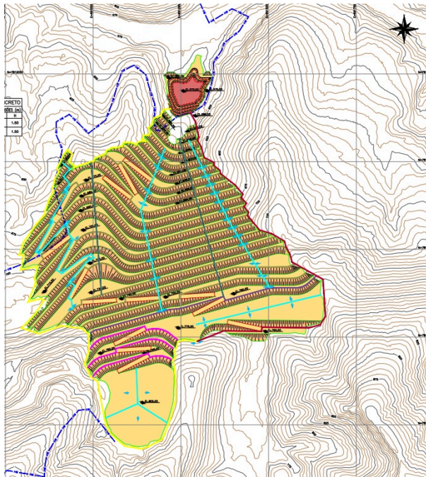
Figura 2: Visão em planta da Pilha de Disposição de Estéril PDE-11, integrante da Planta Industrial da Mina do Andrade
