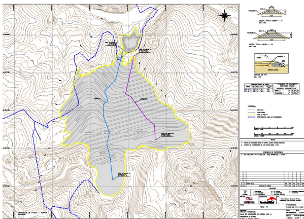
Figura 3: Planta baixa dos Drenos de Fundo DF-11.01 (N-28) e DF-11.02 integrantes do Sistema de Drenagem Interna da PDE-11 da Mina do Andrade
