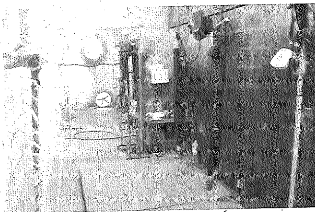
Foto 3: Área do used (envelhecimento das peças).
