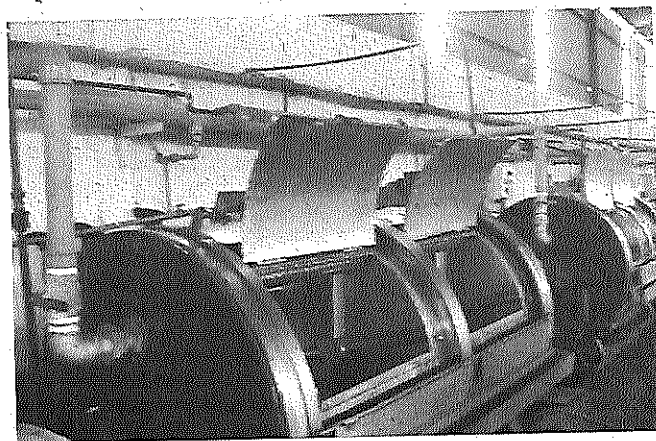
Foto 1: Área de lavagem, tingimento e amaciamento de peças.
