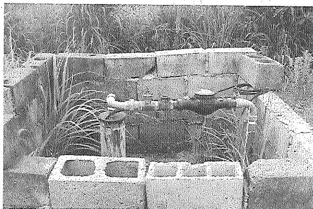
Foto 19: Poço de captação de água com medidor de vazão.
