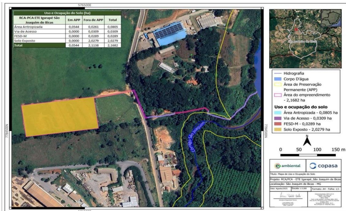
Imagem 01- Área de instalação da ETE Igarapé/São Joaquim de Bicas
