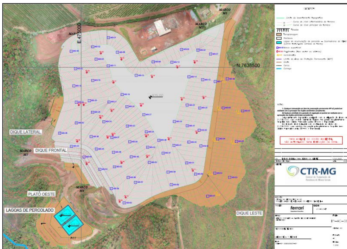
Figura 26 – Locação final da rede de instrumentação geotécnica do aterro Classe II. Fonte: Estudos ambientais.
