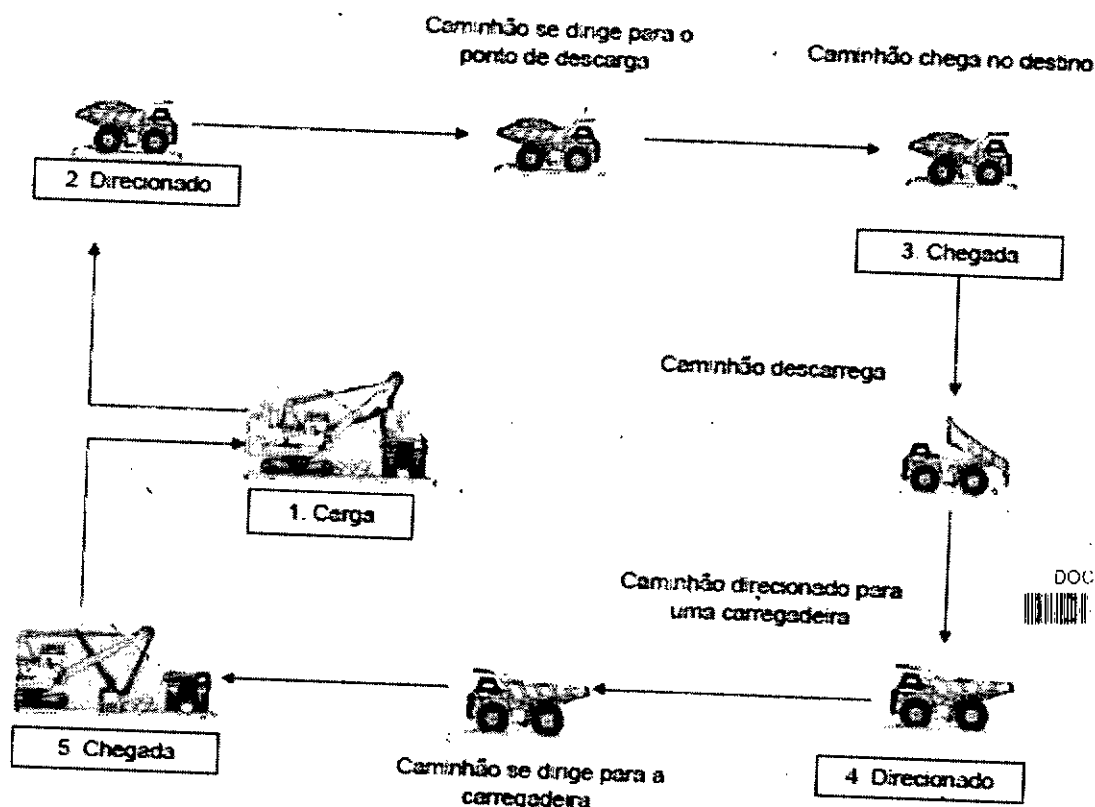
Figura 2: Diagrama do processo de carregamento e transporte.
