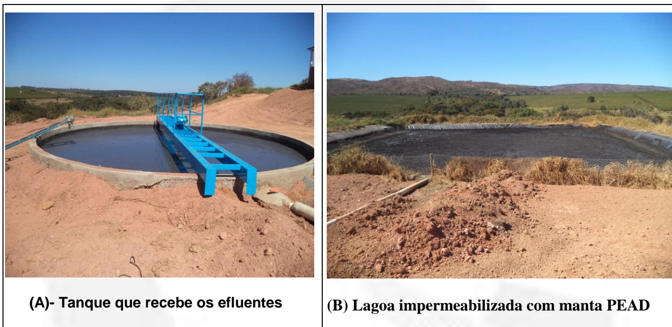
Figura 01 – Sistema de tratamento de efluentes
