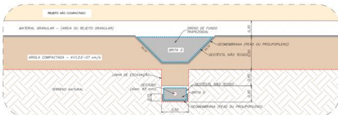
Figura 5 Detalhe- impermeabilização dos dispositivos de drenagem interna Fonte: EIA, 2024
