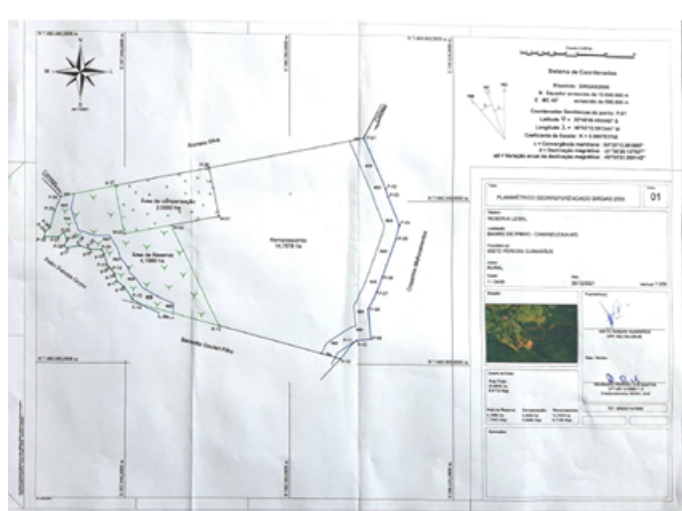
Figura 14: Planta planialtimétrica do Sítio Paraíso, Bairro do Pinho, município de Camanducaia/MG.
