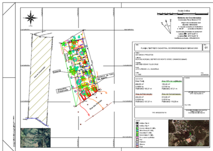
Figura 3: Planta planialtimétrica do Lote 02J, Quadra A, situado à Rua das Acácias, Loteamento Balneário Monte Verde, Distrito de Monte Verde, Camanducaia/MG.
