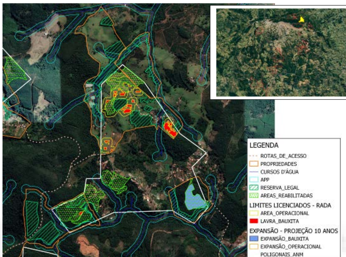
FIGURA 8 – Imagem aérea da Minas Alto do Selado e Colina. Fonte: Autores.
