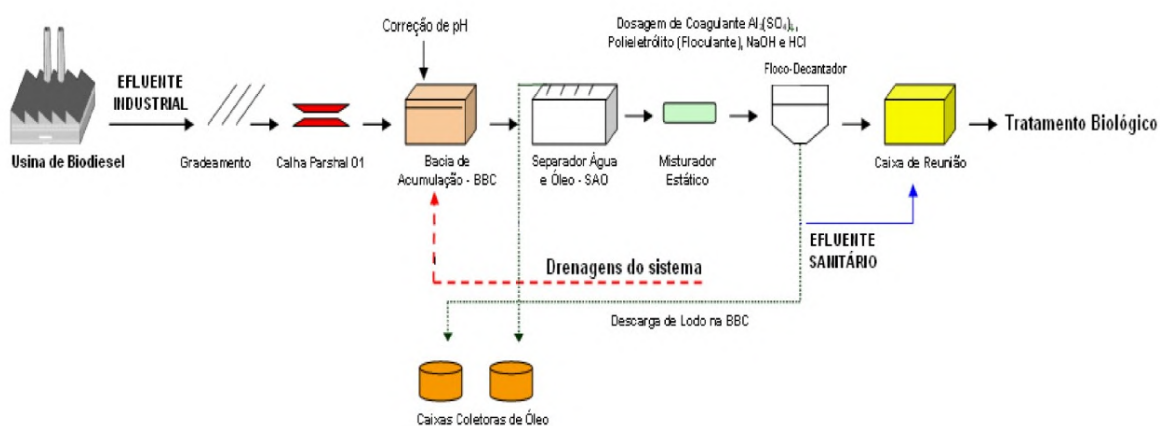
Figura 5 – Fluxograma do tratamento físico-químico do efluente industrial
