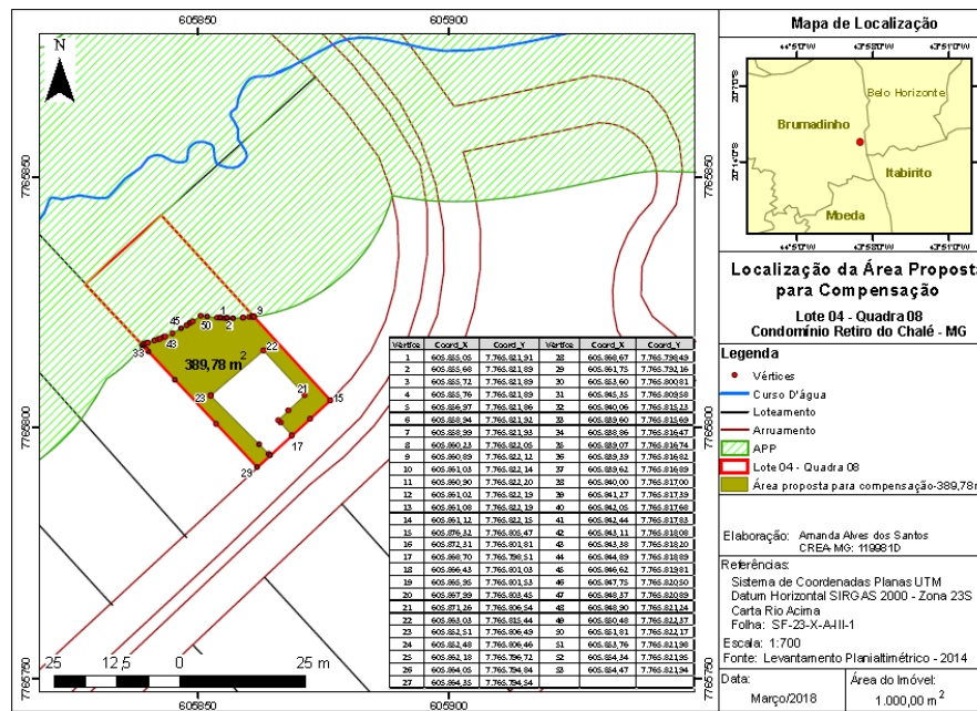
Figura 02 – Planta ilustrando a área de compensação. Fonte PECF 2017
