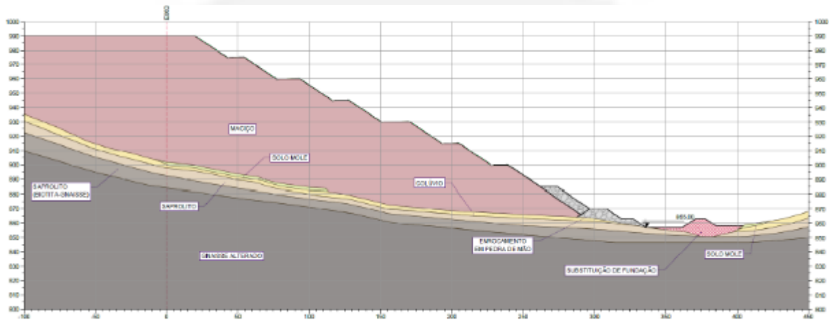
Figura 5 – Perfil topográfico da pilha. Fonte: Projeto Executivo.
