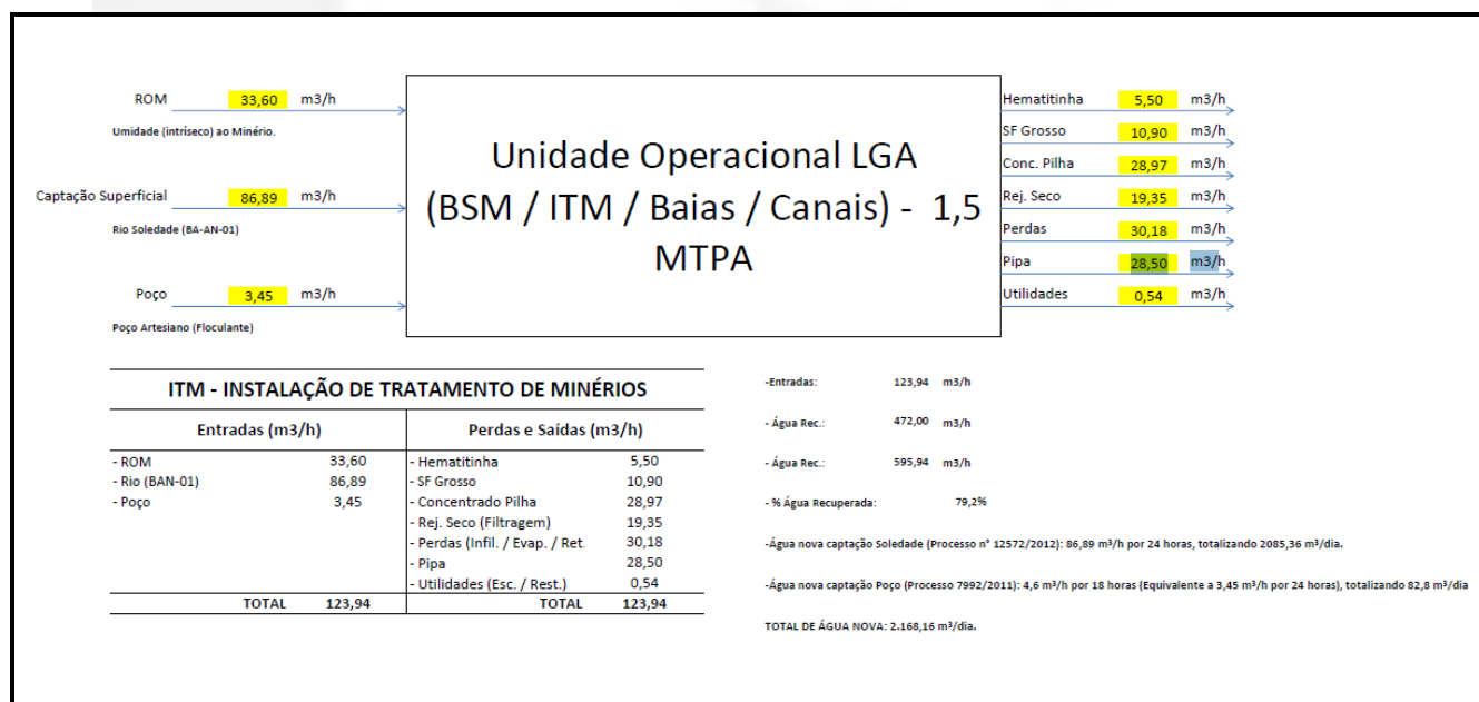
Figura 4 – Balanço Hídrico.
