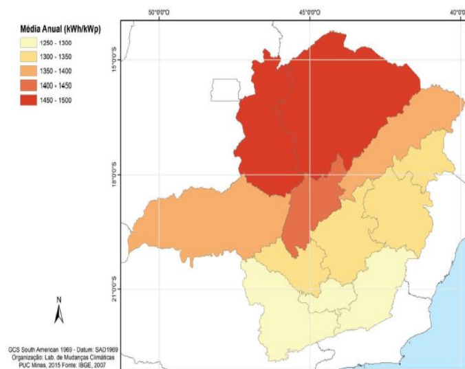
Potencial Solar
