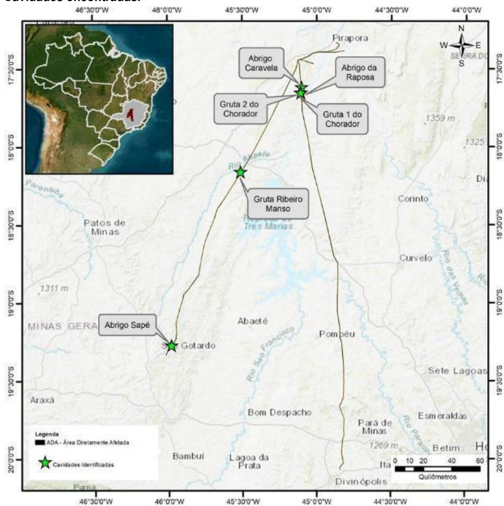
Figura 36. Cavernas encontradas.
