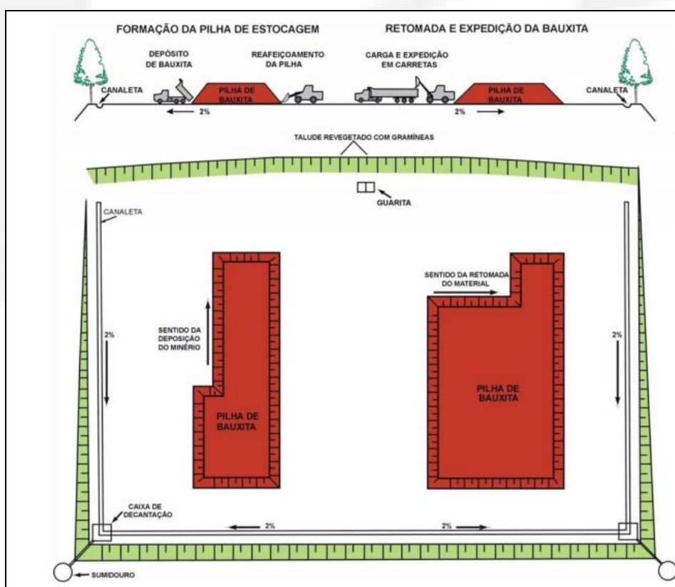
FIGURA 45 – Croqui do pátio de estocagem de minério da CGM.
