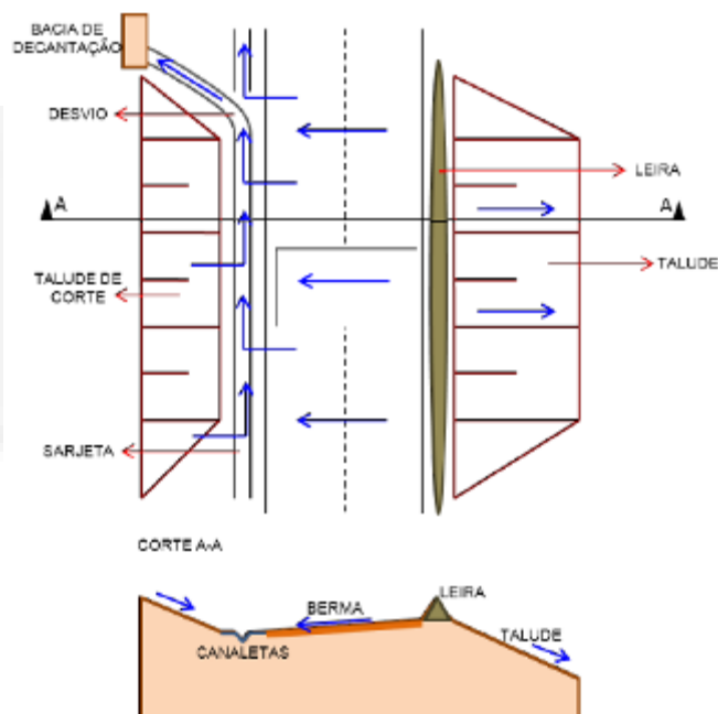
FIGURA 59 – Esquema do sistema de drenagem de águas pluviais. Fonte: Estudos ambientais.
