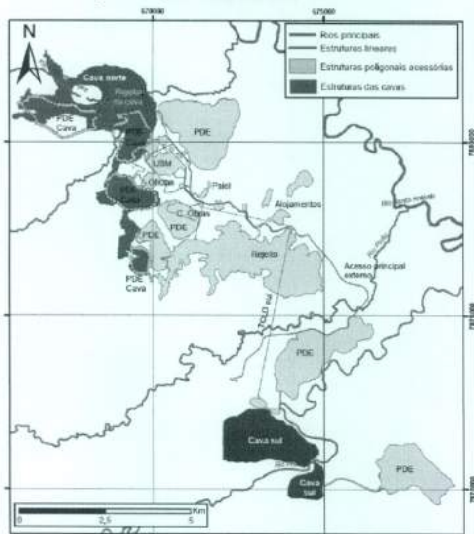
Figura 1-10 – Layout das estruturas da alternativa locacional 4
