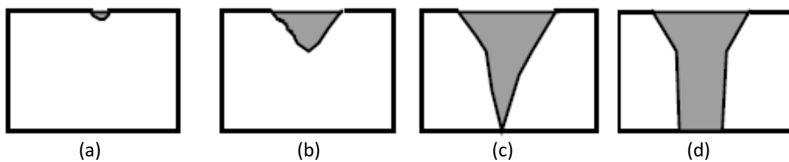
Figura 42: Evolução da falha de uma barragem causada por galgamento ou overtopping em vista esquemática frontal da barragem (adaptado de Johnson e Illes, 1976).
