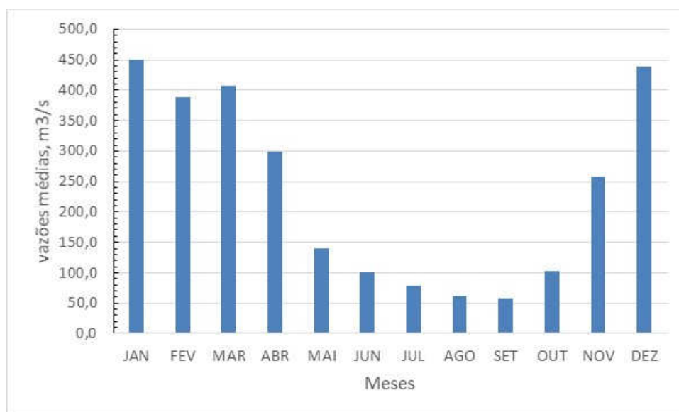
Figura 92: Variação sazonal do posto 43880000
