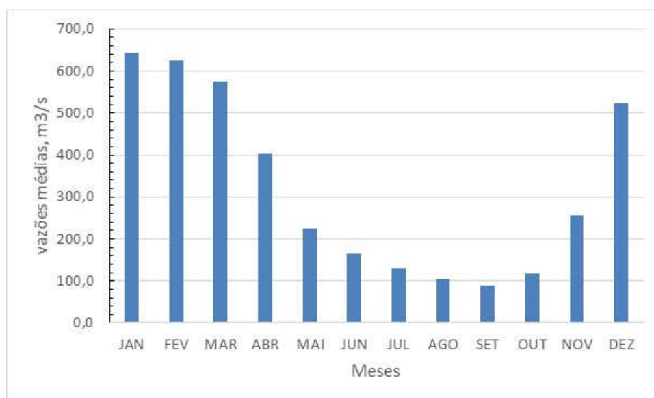
Figura 88: Variação sazonal do posto 42690000
