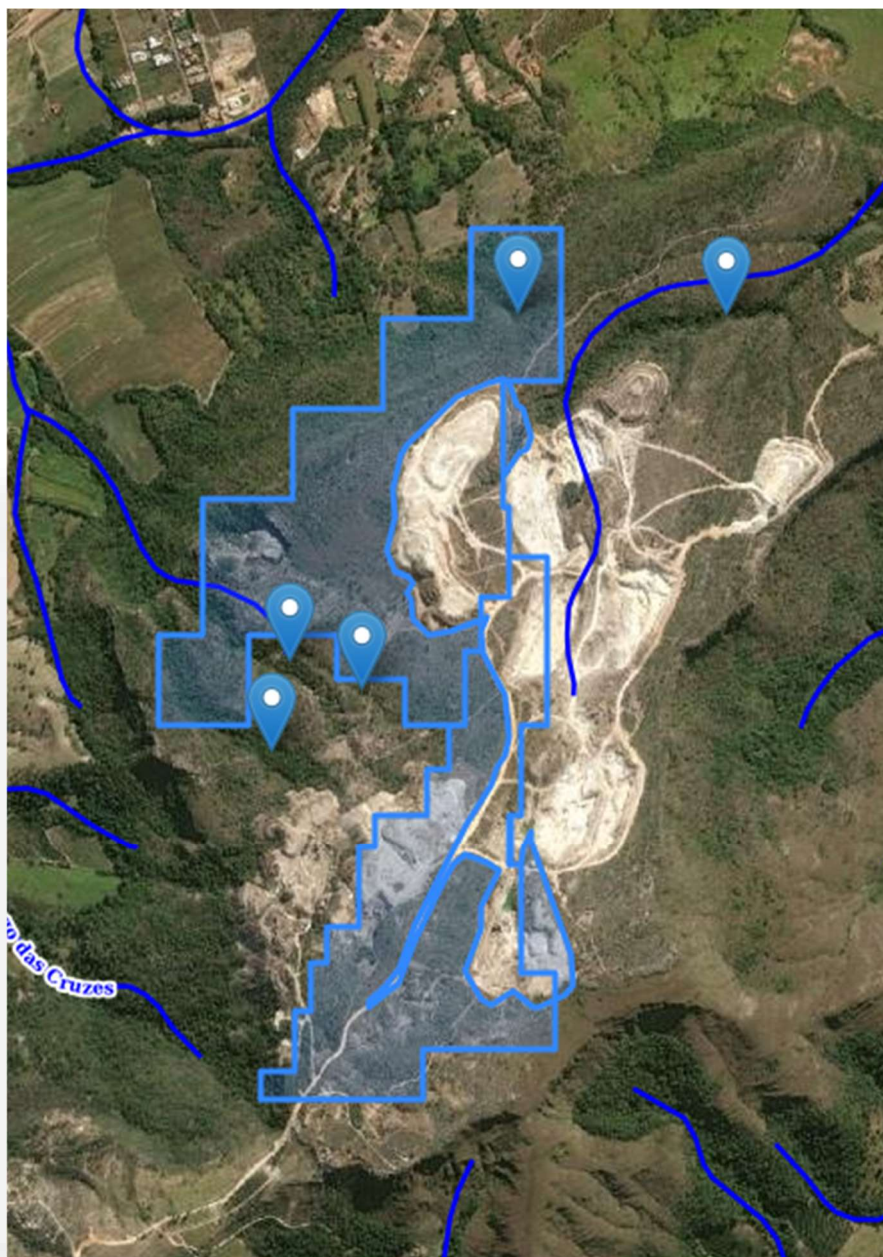
Figura 4 – Camada ortofotoretos da bacia do rio Grande e pontos da grotta seca sobrepostos a ADA e ANM da Pedras São Lucas. Fonte: IDE-Sisema.
