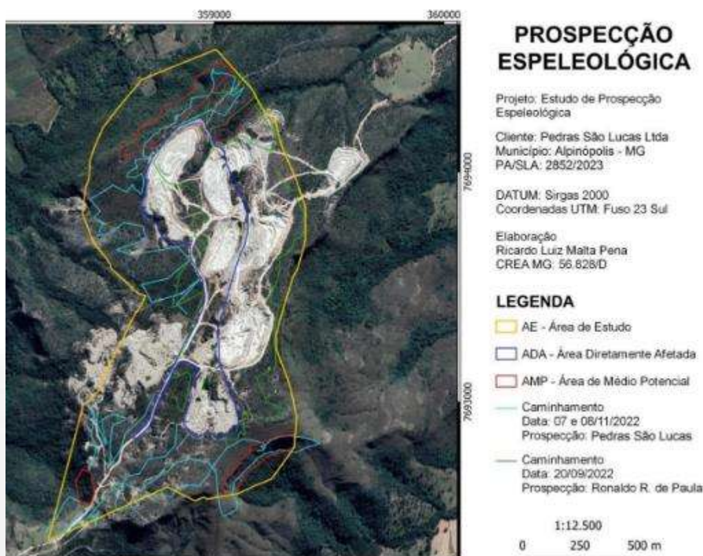
Figura 3 – Prospeção espeleológica. Fonte: SEI 79222643.
