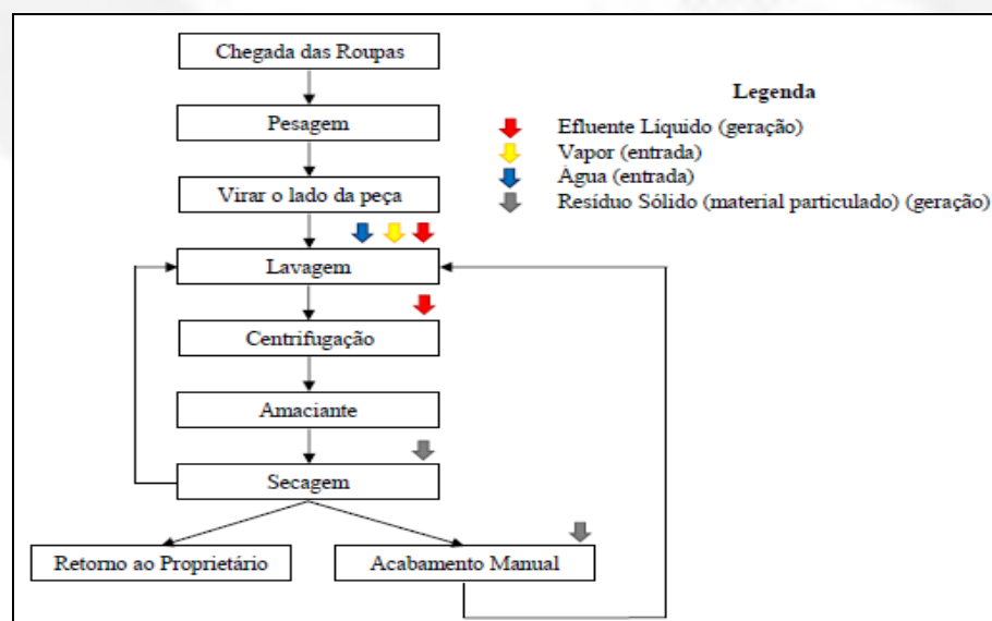
FIGURA 2: Fluxograma do processo produtivo.
