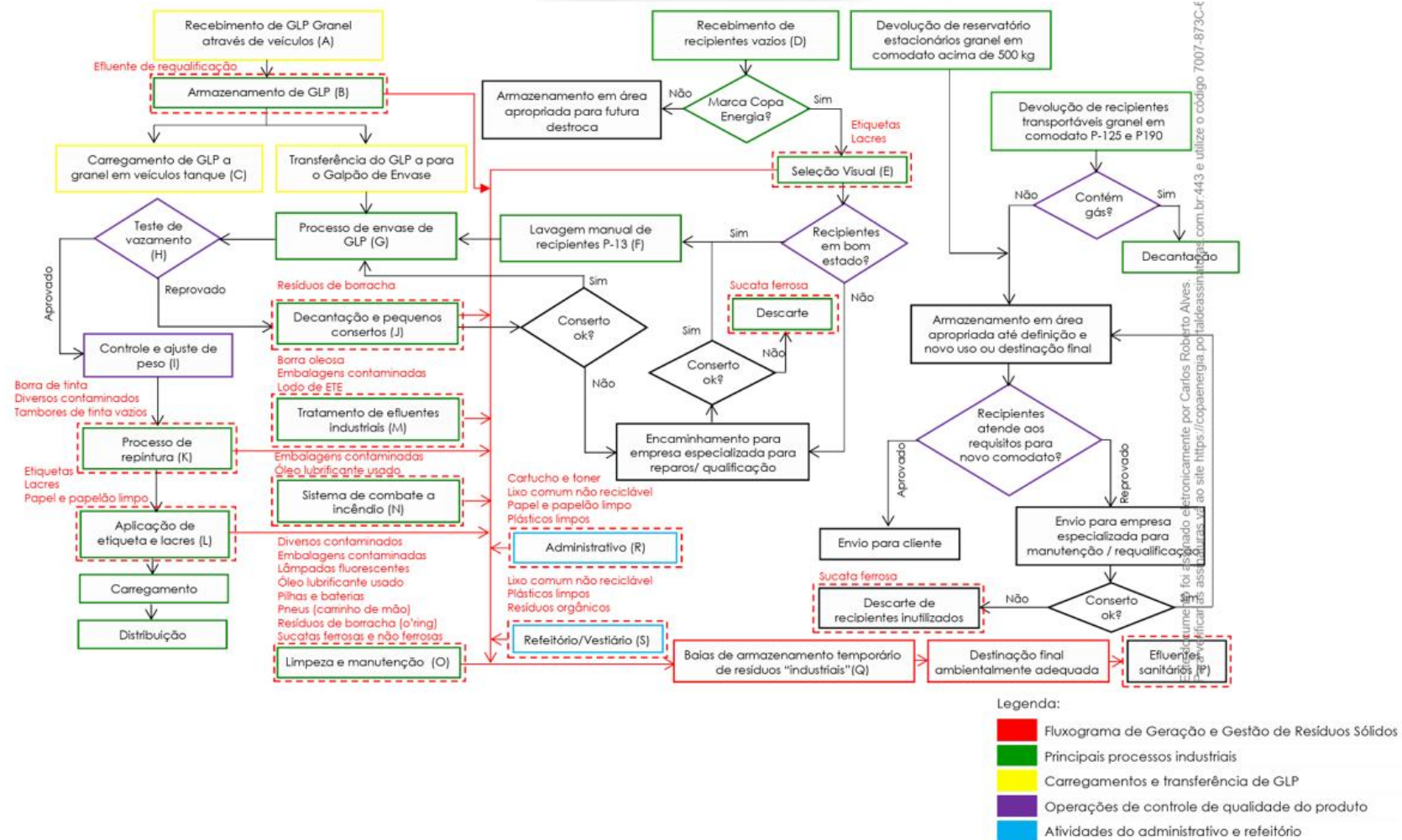
Figura 04: Fluxograma de geração e gestão dos resíduos sólidos gerados no Centro Operativo da Copa Energia em Uberlândia
