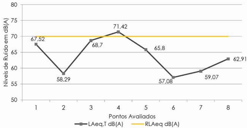
Figura 08: Níveis de pressão sonora específicos em cada ponto avaliado e limite estabelecido pela Lei Estadual nº 10.100/1990 para período diurno Fonte: RCA (p. 23)
