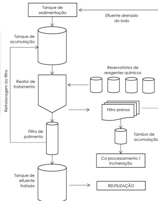
Figura 03: Fluxo de tratamento dos efluentes industriais na ETEI do Centro Operativo Fonte: RCA (p. 26)
