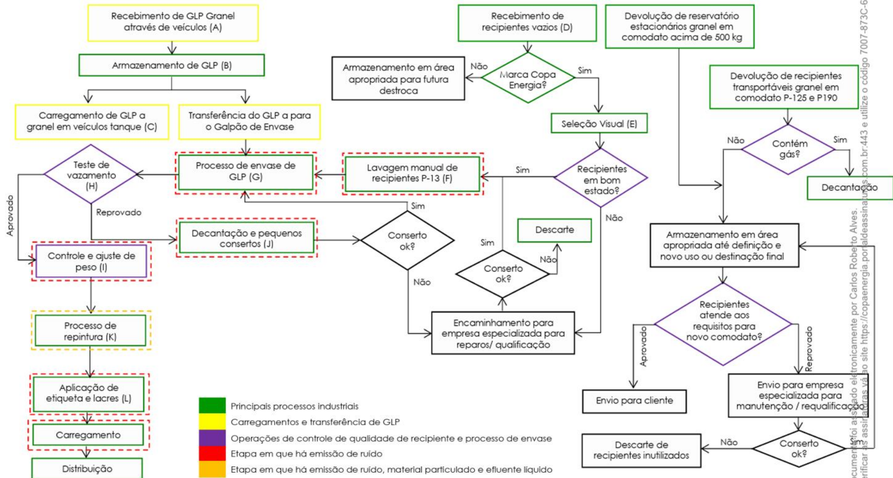
Figura 02: Fluxograma do processo produtivo do Centro Operativo da Copa Energia em Uberlândia Fonte: Adaptado do RCA (p. 14)
