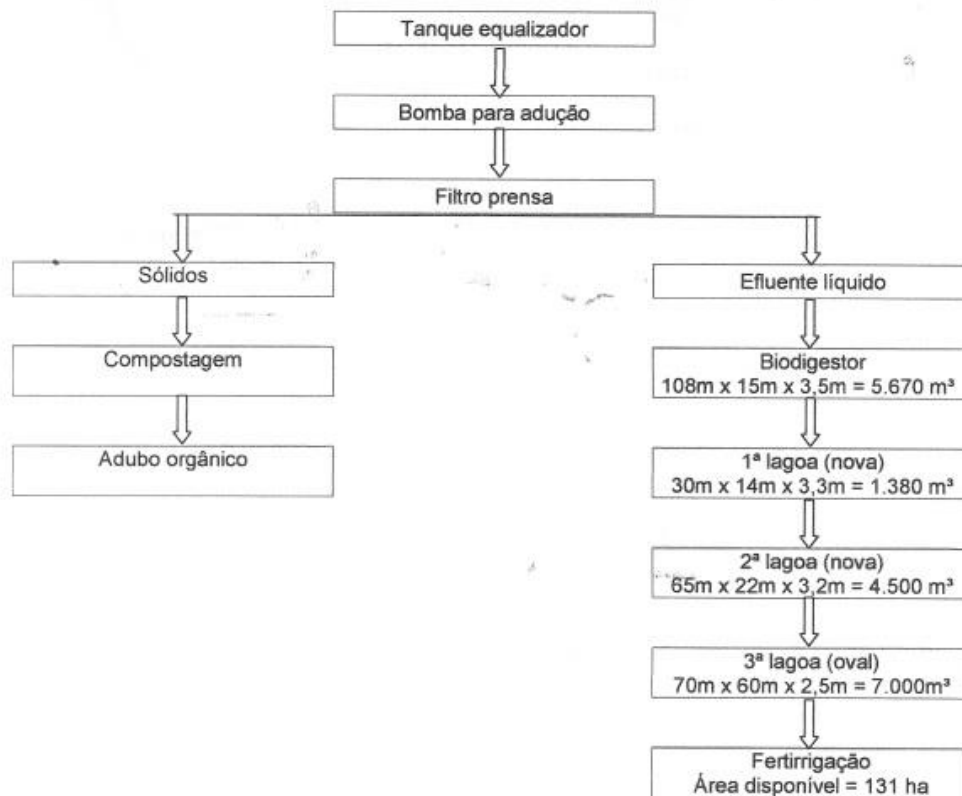
Fluxograma do Sistema de Tratamento de Efluentes após adequação:
