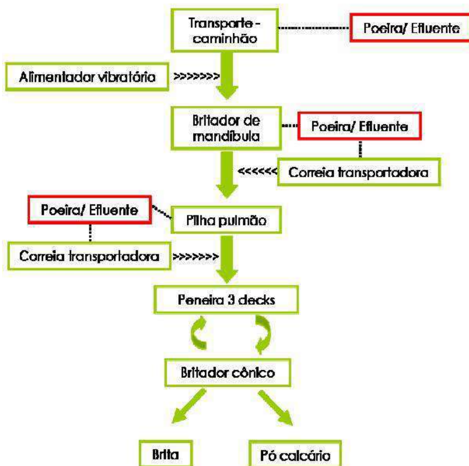
Figura 4- Fluxograma do processo de beneficiamento do basalto. Fonte: RCA BRITAGEM TRÊS IRMÃOS LTDA. (2025)
