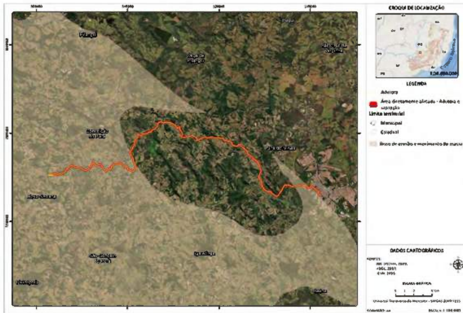
Figura 2.4. Mapa risco de erosão e movimento de massa
