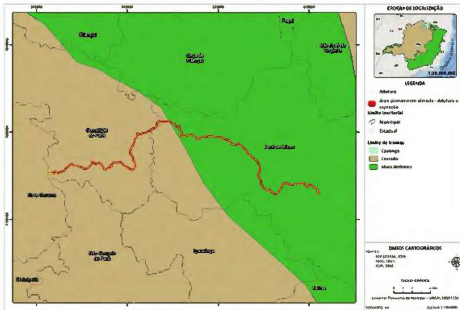
Figura 2.13. Limite dos biomas (IBGE 2004); Limite do bioma Mata Atlântica – Lei nº11.428/2006
