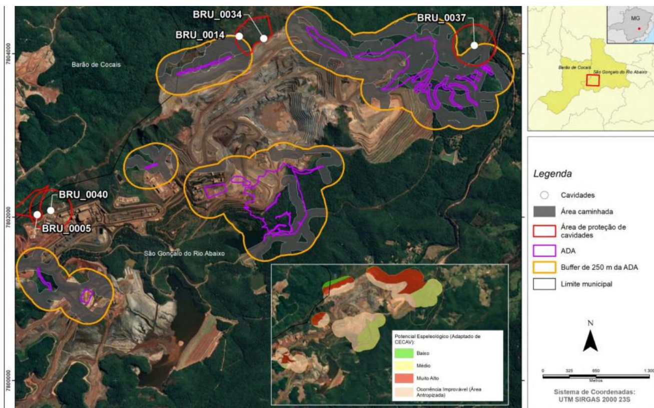
Figura 23 – Caminhamento e potencial espeleológico na área de ampliação. Fonte: EIA
