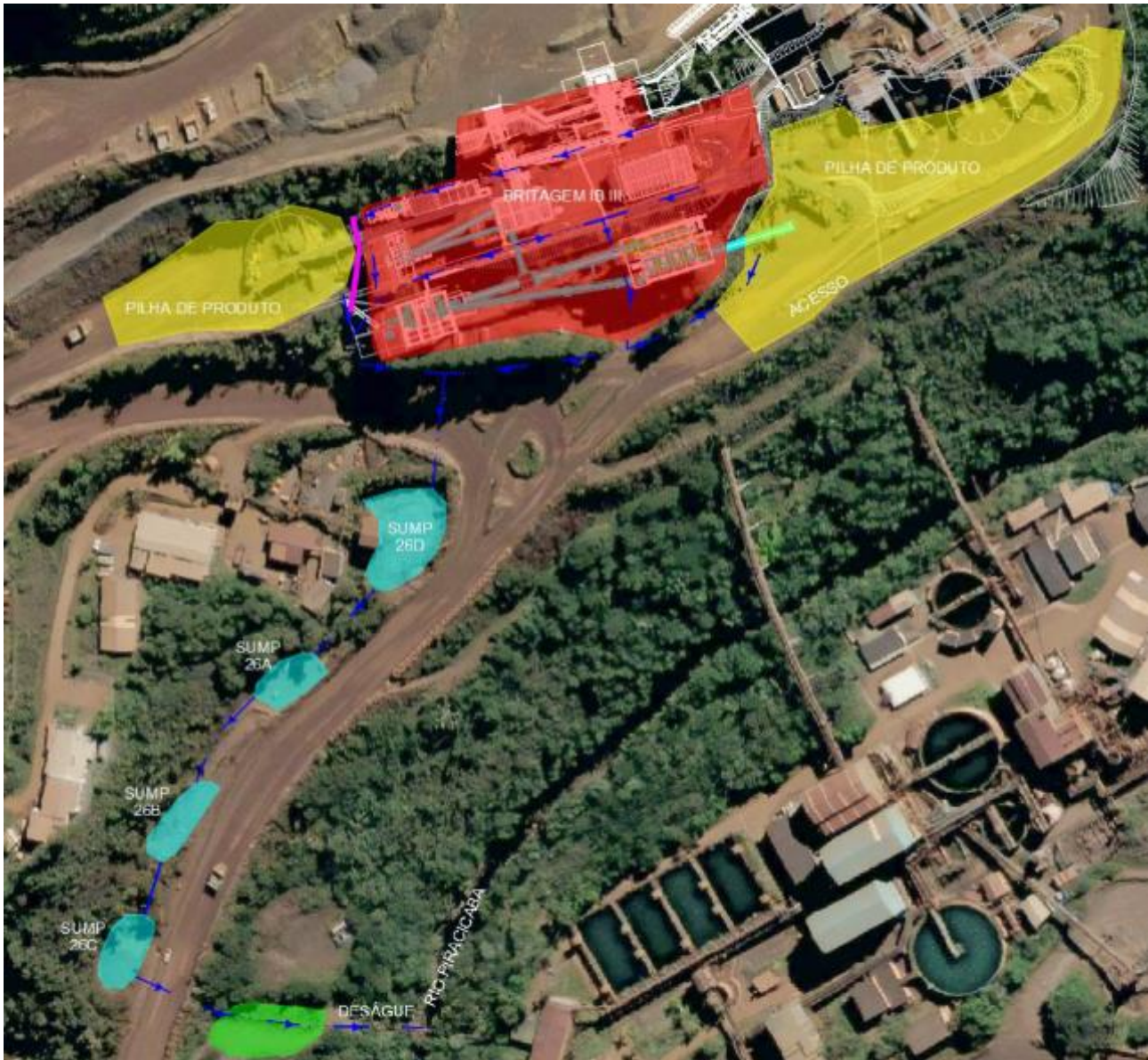
Figura 12. Sistema de Drenagem existente na área da Britagem da IB-III.
