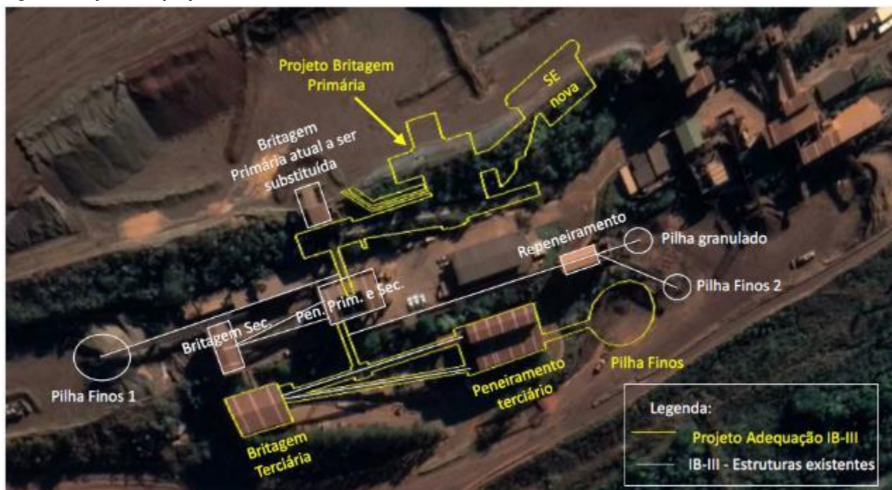
Figura 7. Layout do projeto da Usina IB-III.
