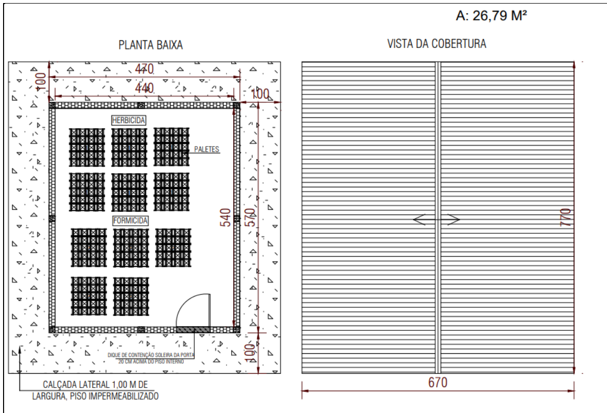
Figura 05: Galpão de armazenamento de agrotóxico.
