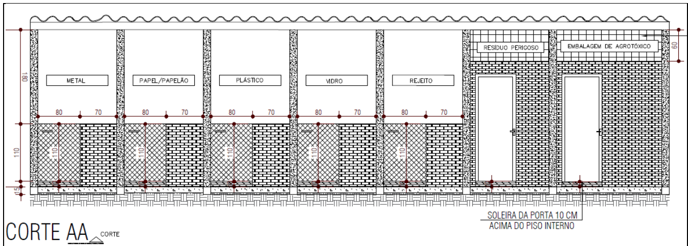
Figura 34: Central de Armazenamento Temporária de Resíduos Sólidos.
