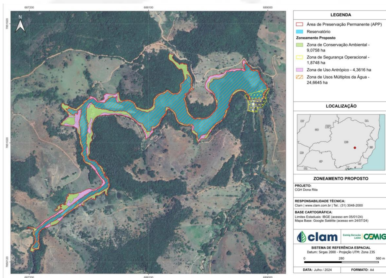
Figura 14: Zoneamento proposto para a CGH Dona Rita.
