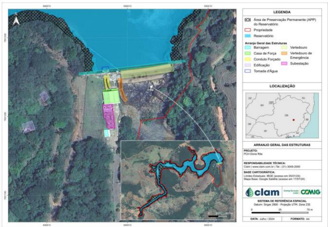
Figura 2: Arranjo físico do empreendimento. Fonte: RADA, 2024.
