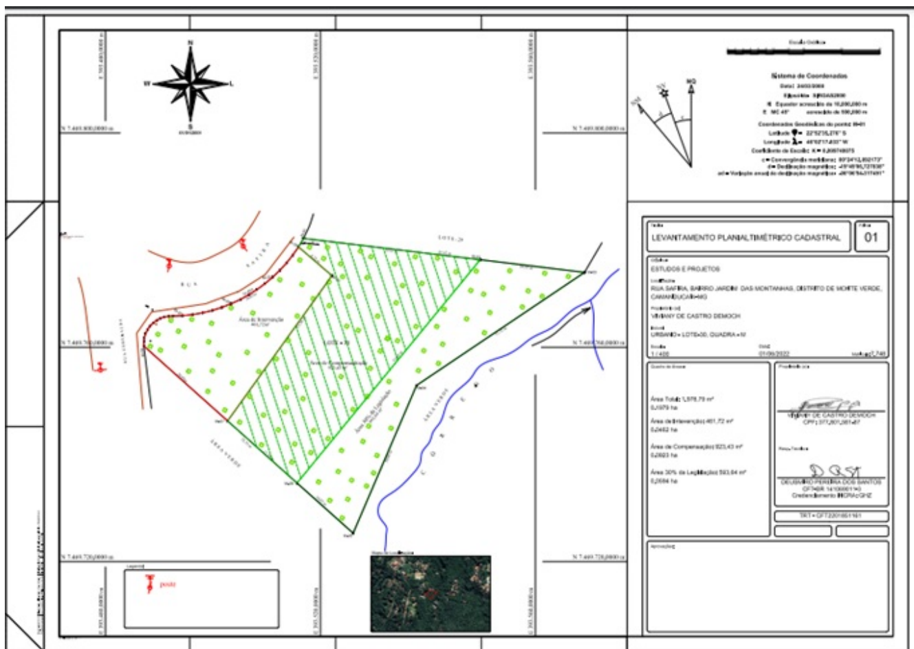
Figura 3: Planta planialtimétrica do Lote 30 da Quadra M, Loteamento Recanto do Selado, Distrito de Monte Verde, Camanducaia/MG.
