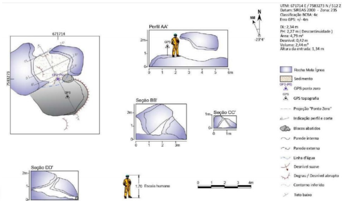
Figura 12 - Mapa topográfico da caverna MTB-0001. RCA, Clam Meio Ambiente, 2022.
