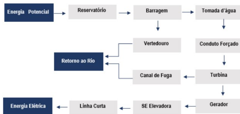
Figura 6-2. Fluxograma do processo produtivo de geração de energia. Fonte: CEMIG, 2022. Elaborado por Clam, 2022.
