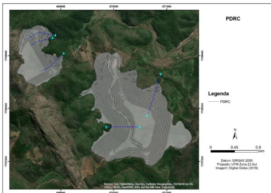
Figura 7- Arranjo geométrico da PDER C. Fonte: EIA
