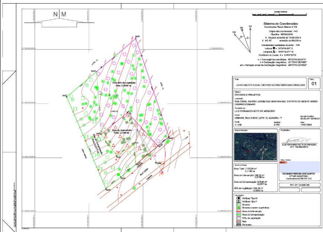
FIGURA 03: Planta planialtimétrica do Lote nº. 16 da quadra T, situado à Rua Cisne no Loteamento Jardim das Montanhas, município de Camanducaia/MG, contemplado neste parecer.
