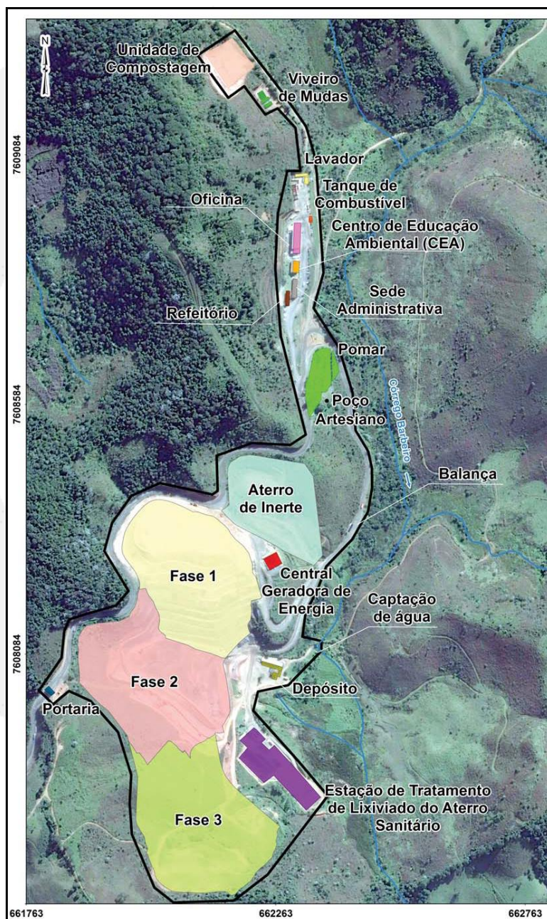
Vista geral das estruturas que compõem a CTRJF.
