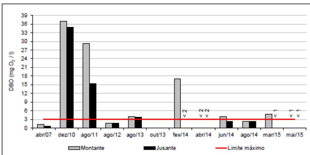
Gráfico 5: BOD analisada no córrego Barbeiro, na ADAE da CTR Juiz de Fora.
