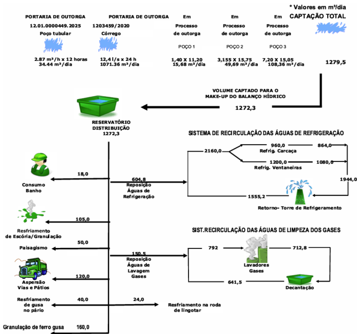
Figura 05: Balanço hídrico apresentado pela empresa no Rima.
