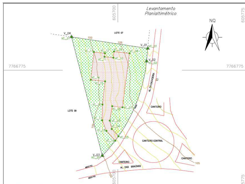
Figura 02 -Planta topográfica ilustrando a área de intervenção/ compensação, dentro do lote. Fonte PECF/2016
