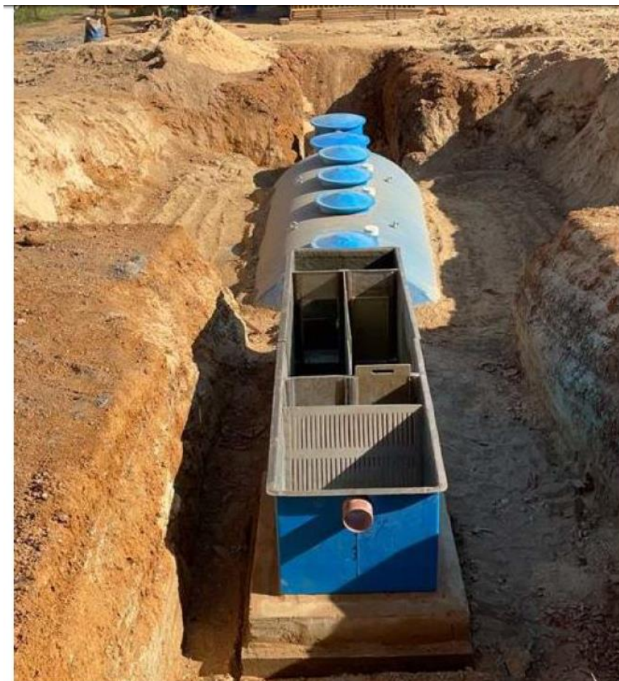
Foto 01: Modelo de estação de tratamento de esgoto que será instalado na Aldeia Indígena.
