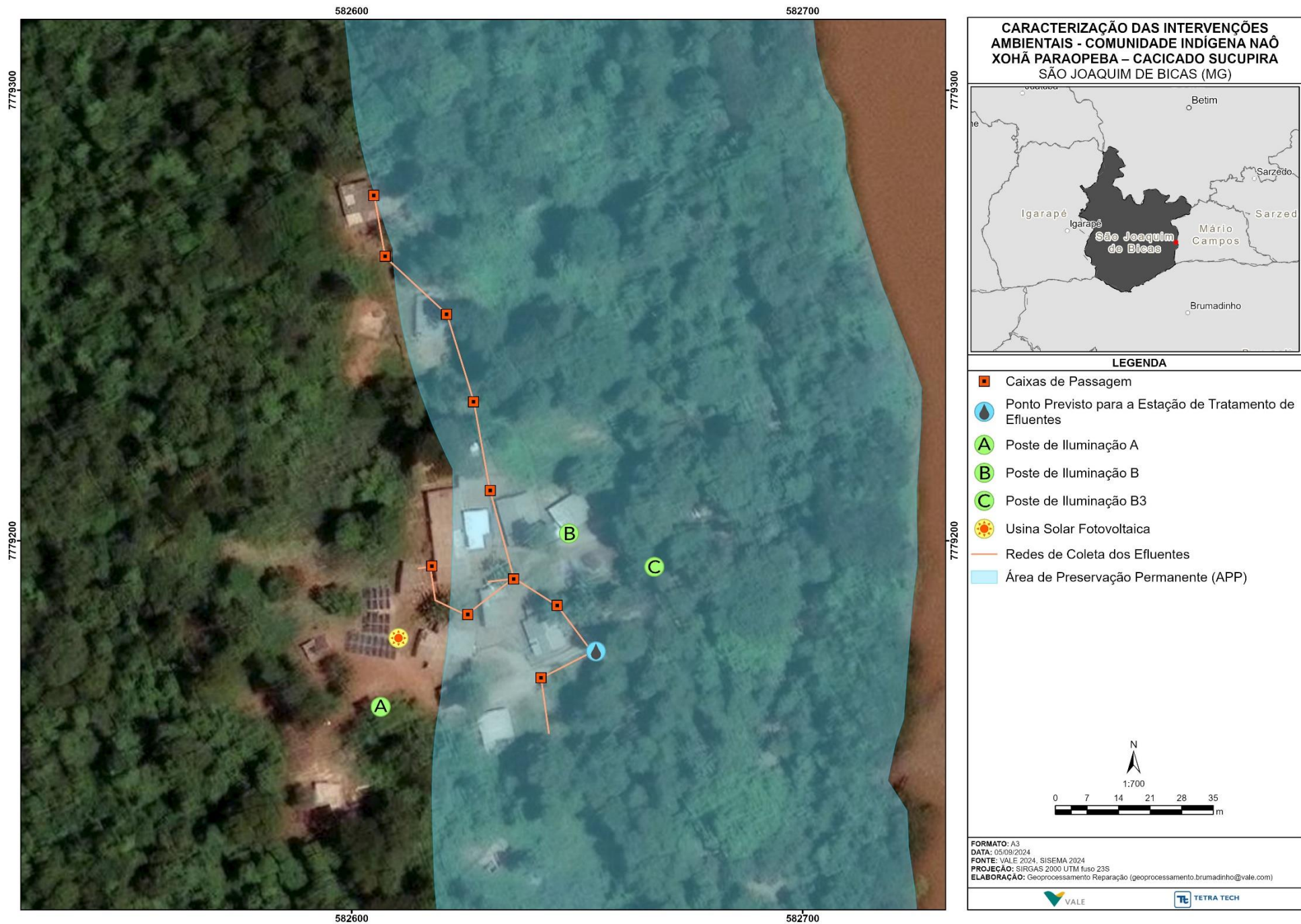
Figura 02: Estruturas previstas para os projetos frente às intervenções ambientais.
