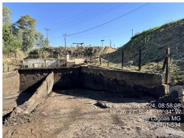
Foto 12: Tanque de decantação de pó de balão, com indícios de retirada recente de material.
