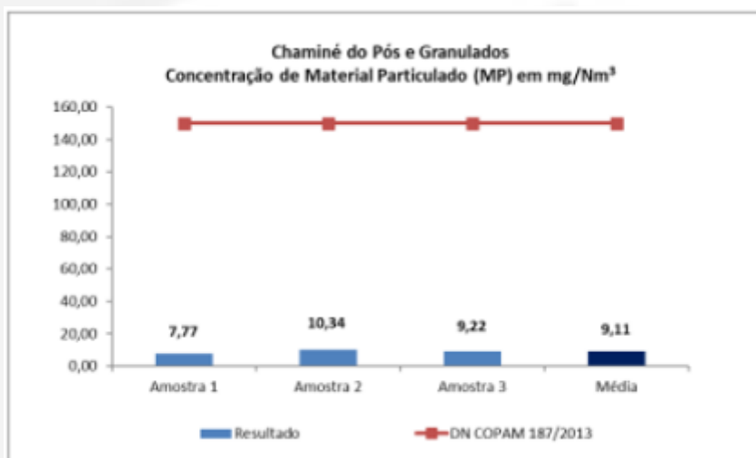
Gráfico 8.5: Monitoramento da chaminé do filtro Pó e Granulados.
