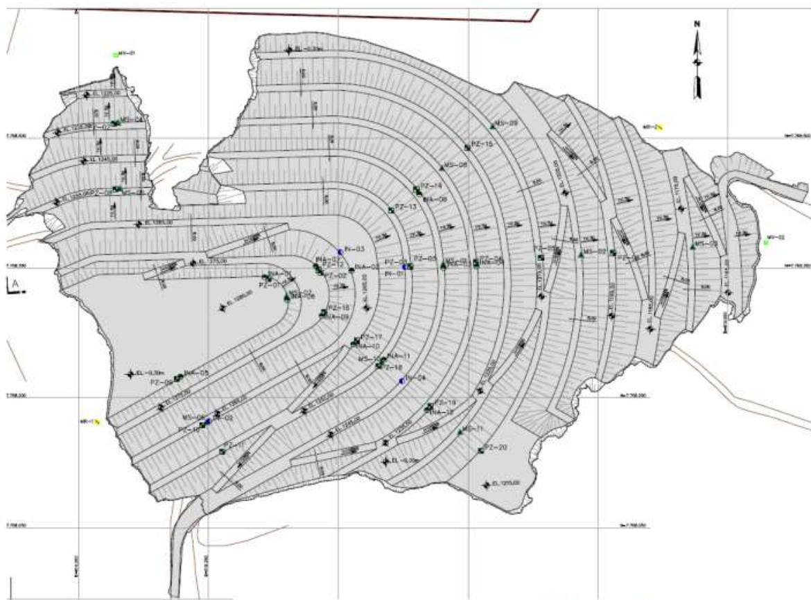
Figura 2.2.8: Plano de Instrumentação da pilha PDER-01
