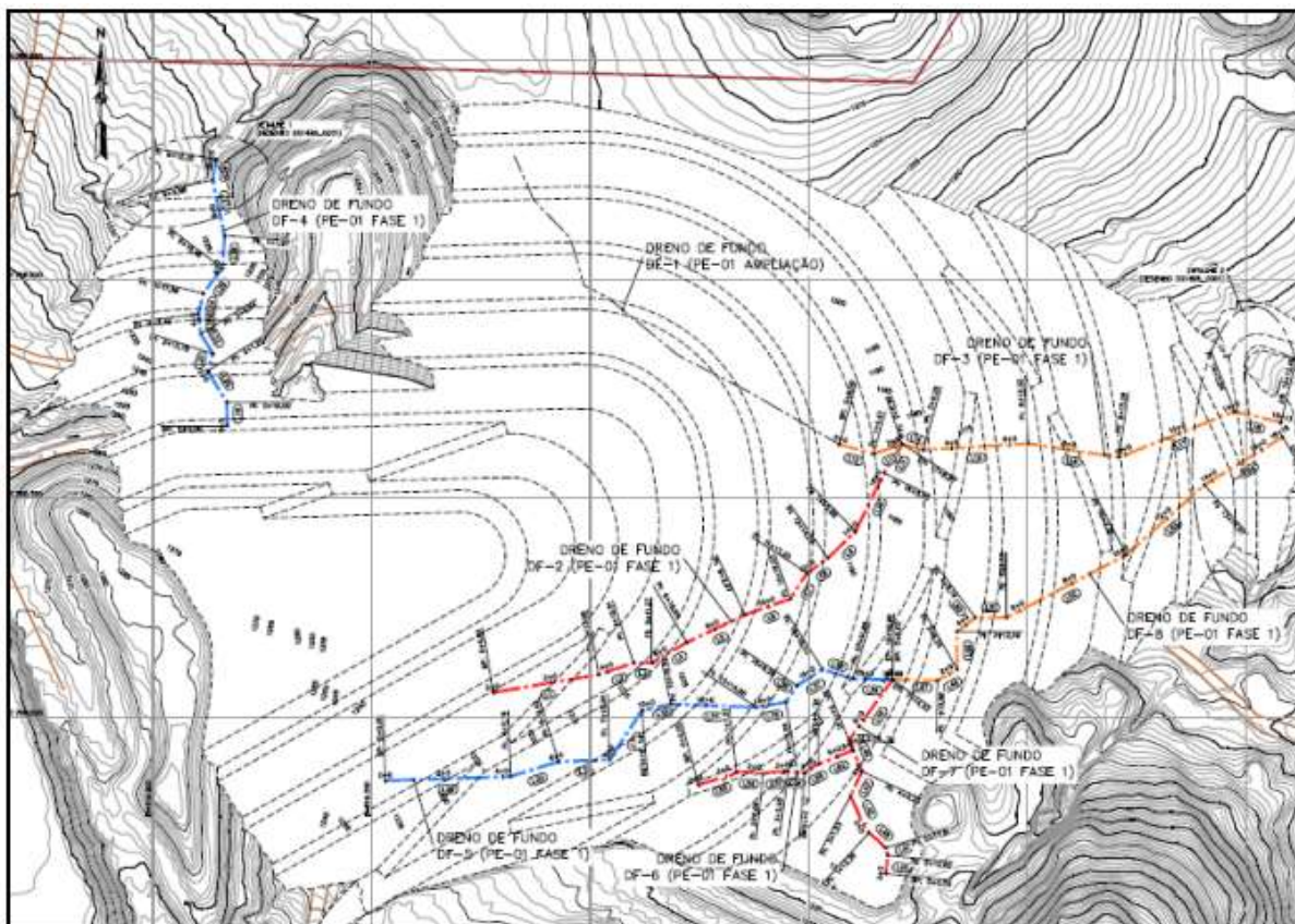
Figura 2.2.7: Arranjo geral de drenagem interna da PDER-01
