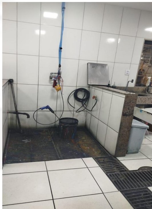
Sistema de drenagem fábrica de tintas
