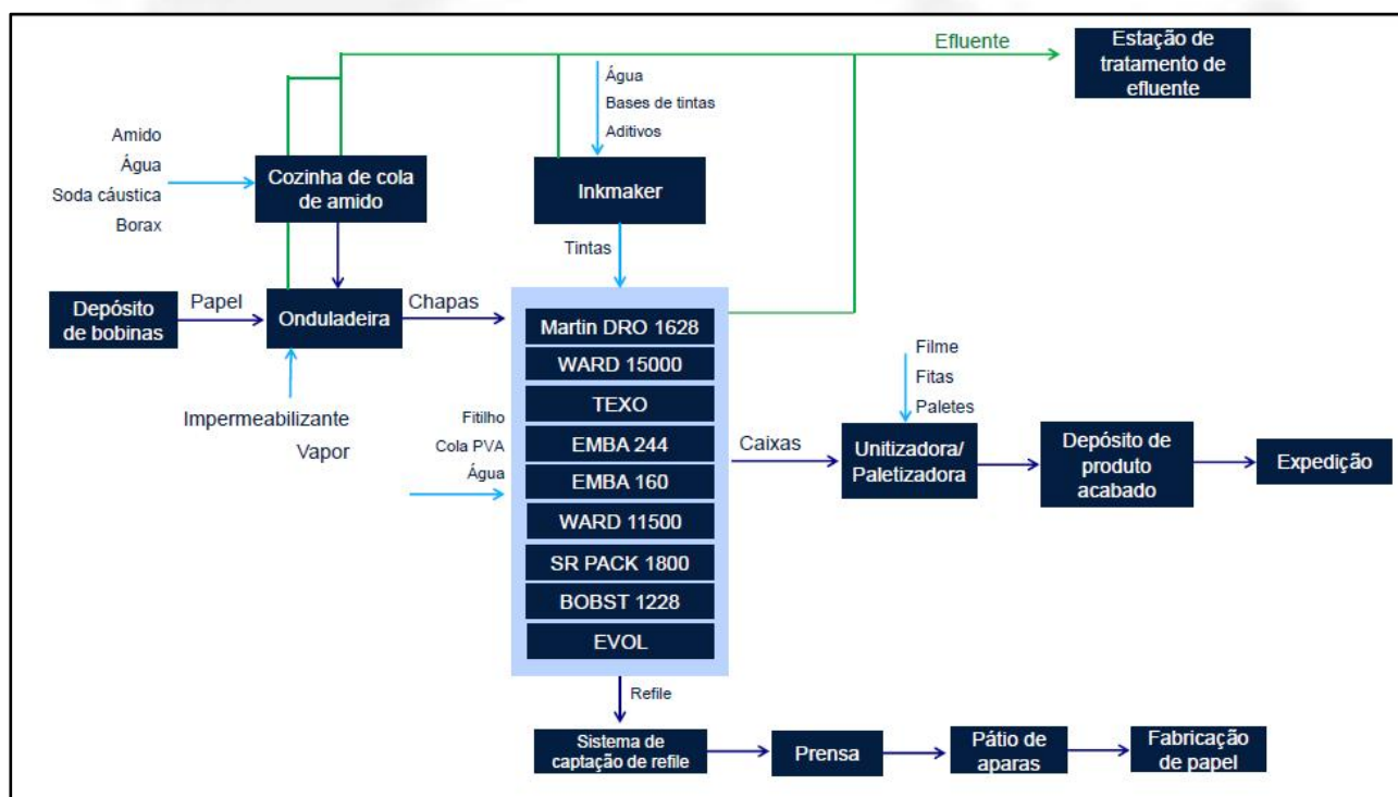
Fluxograma do processo produtivo. Fonte: RCA.
