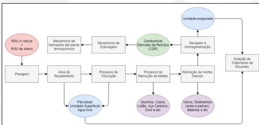
Figura 2: Fluxograma da linha de processamento.
