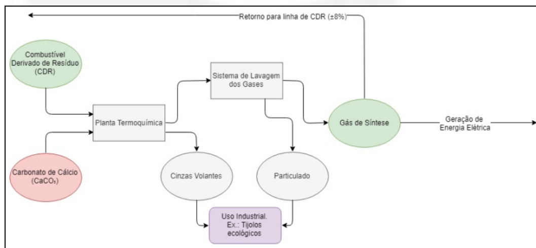
Figura 3: Fluxograma da planta termoquímica.
