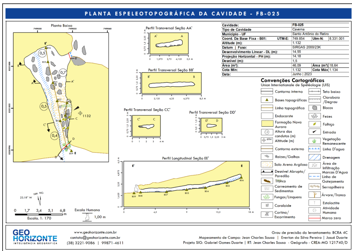
Figura 34: Planta espeleotopográfica – CNS FB-025.
