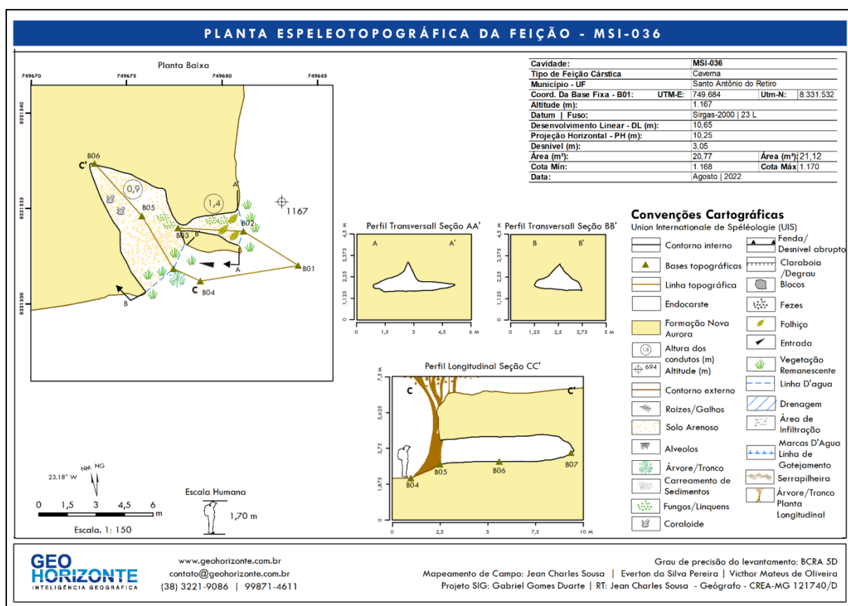
Figura 20: Planta espeleotopográfica – CNS MSI-036.
