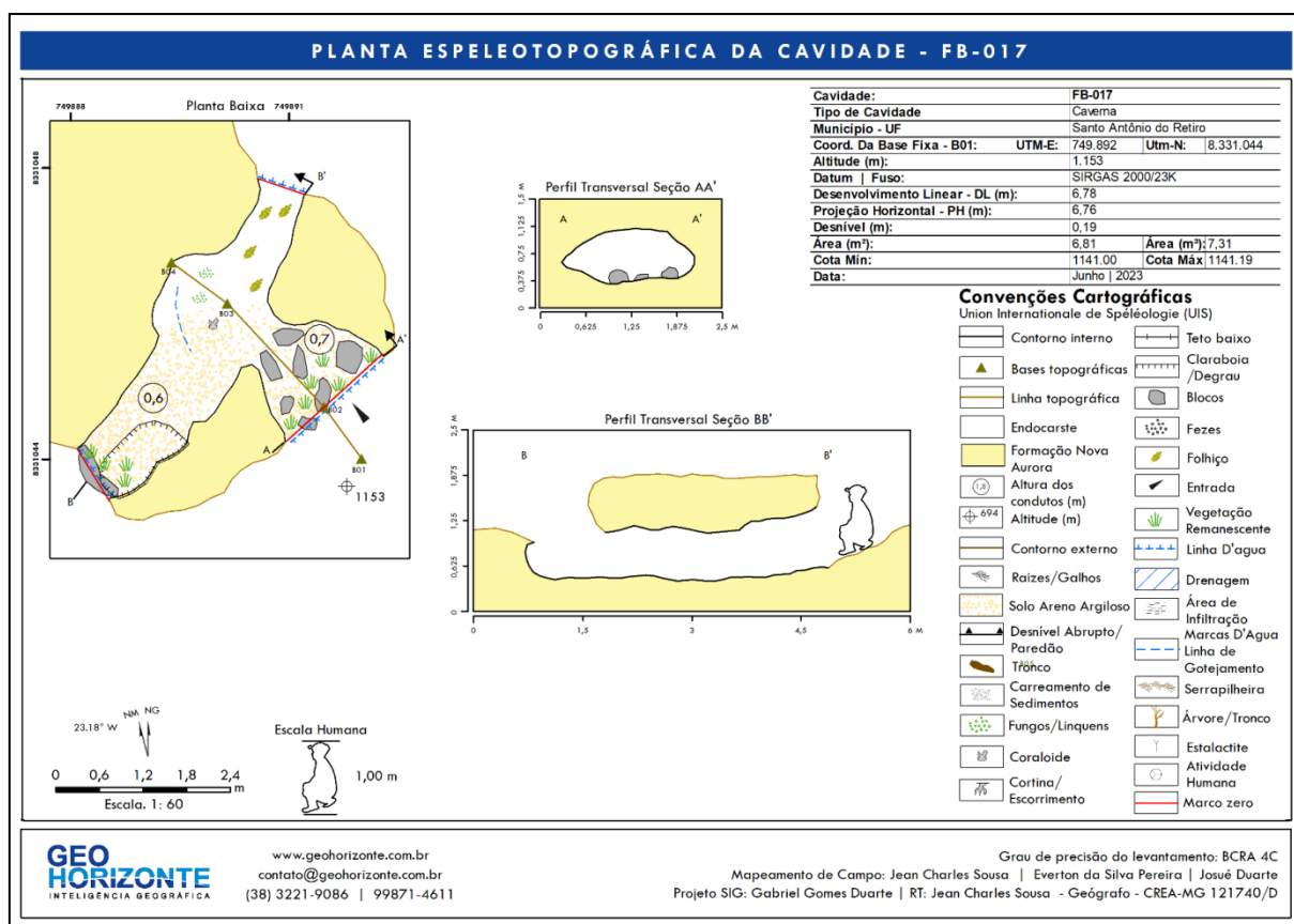
Figura 28: Planta espeleotopográfica – CNS FB-017.
