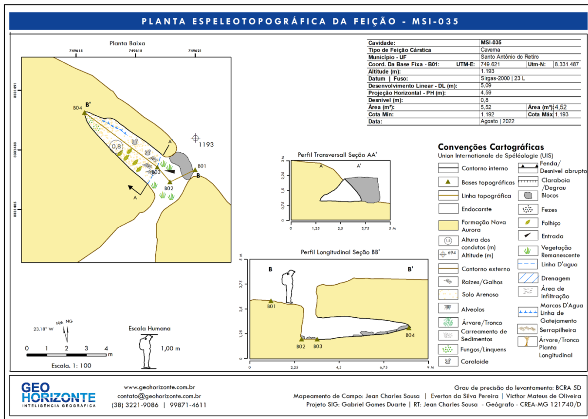
Figura 19: Planta espeleotopográfica – CNS MSI-035.
