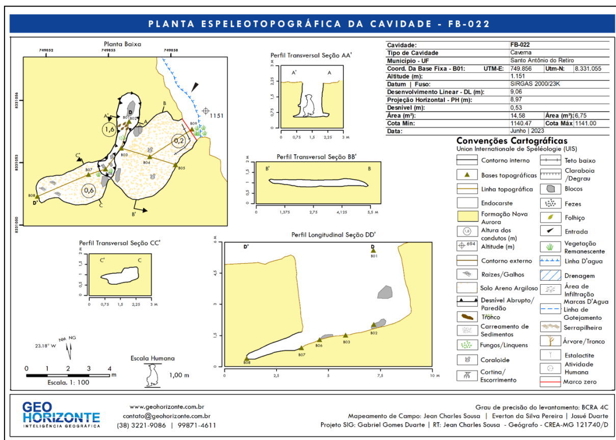
Figura 32: Planta espeleotopográfica – CNS FB-022.
