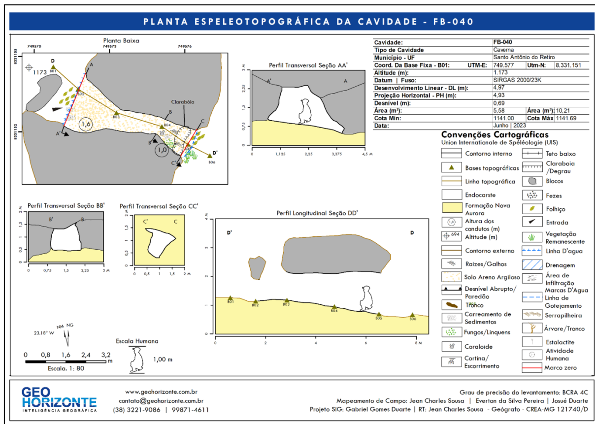
Figura 43: Planta espeleotopográfica – CNS FB-040.
