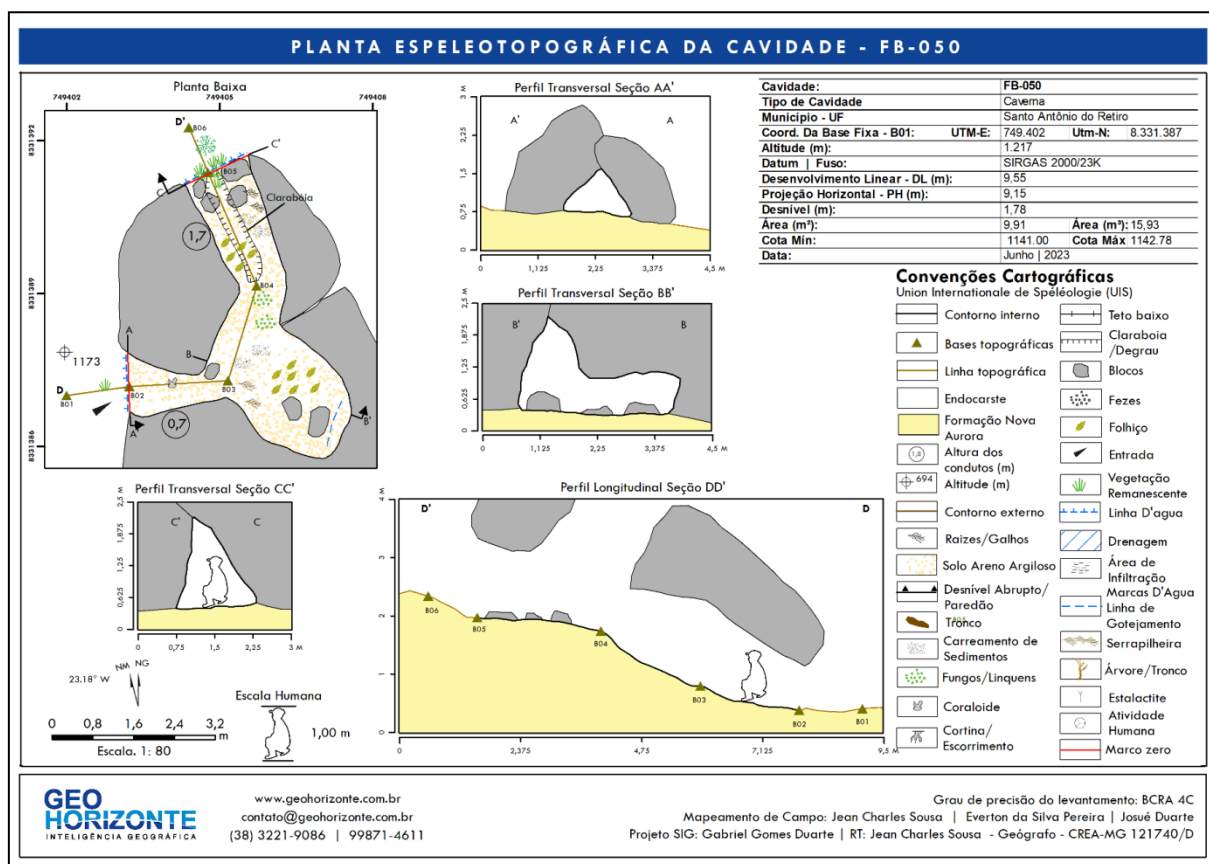
Figura 46: Planta espeleotopográfica – CNS FB-050.
