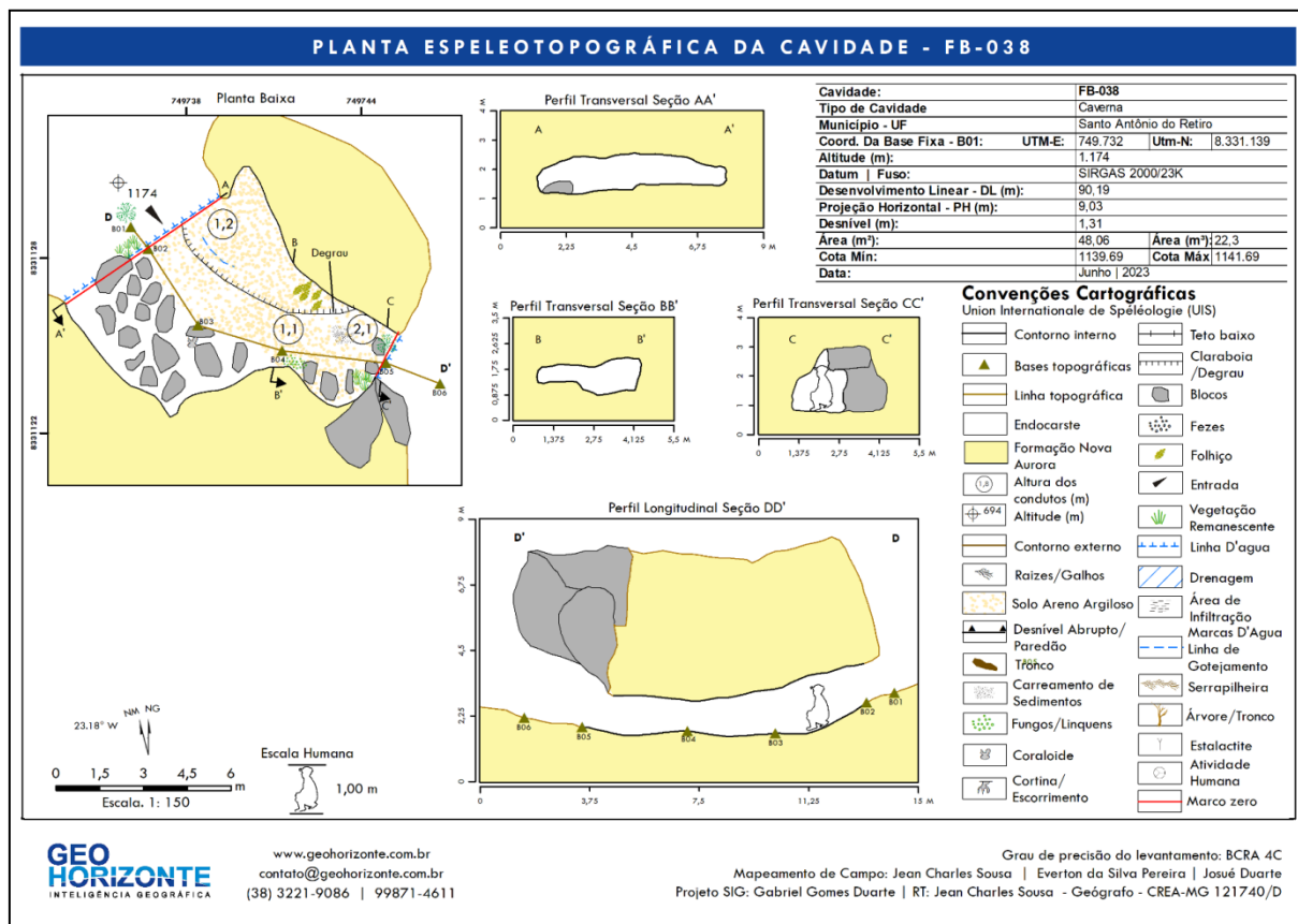
Figura 41: Planta espeleotopográfica – CNS FB-038.
