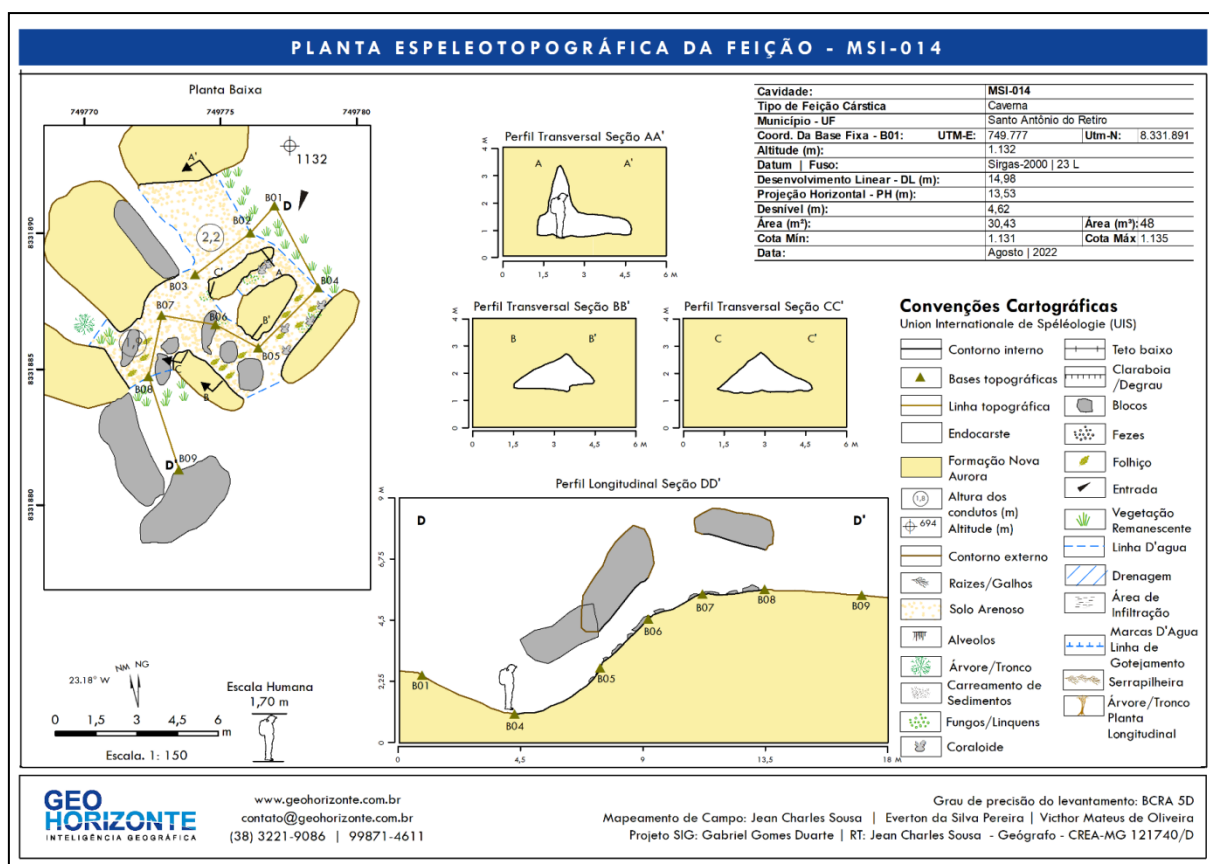
Figura 14: Planta espeleotopográfica – CNS MSI-014.
