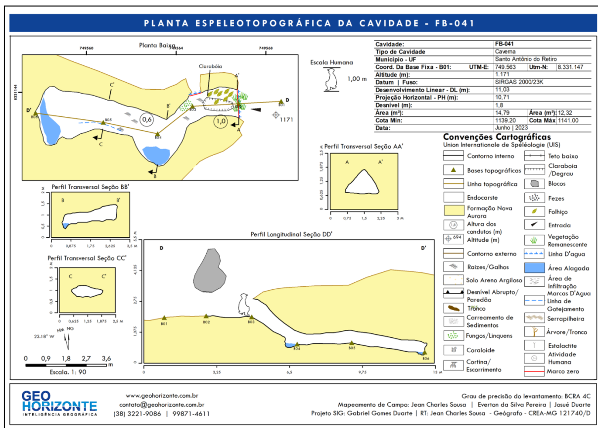
Figura 44: Planta espeleotopográfica – CNS FB-041.
