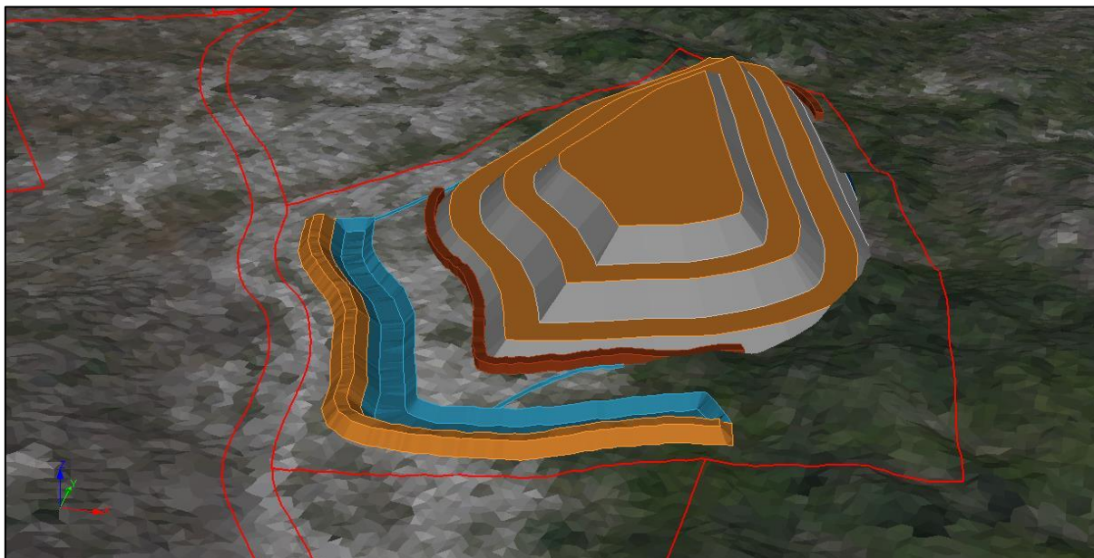
Figura 2: Vista em planta da Pilha de Estéril incluindo localização das seções topográficas.
