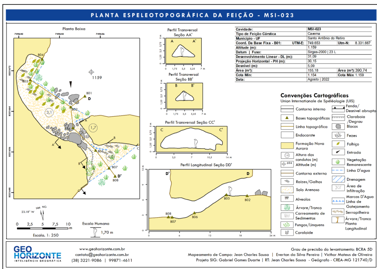
Figura 17: Planta espeleotopográfica – CNS MSI-023.
