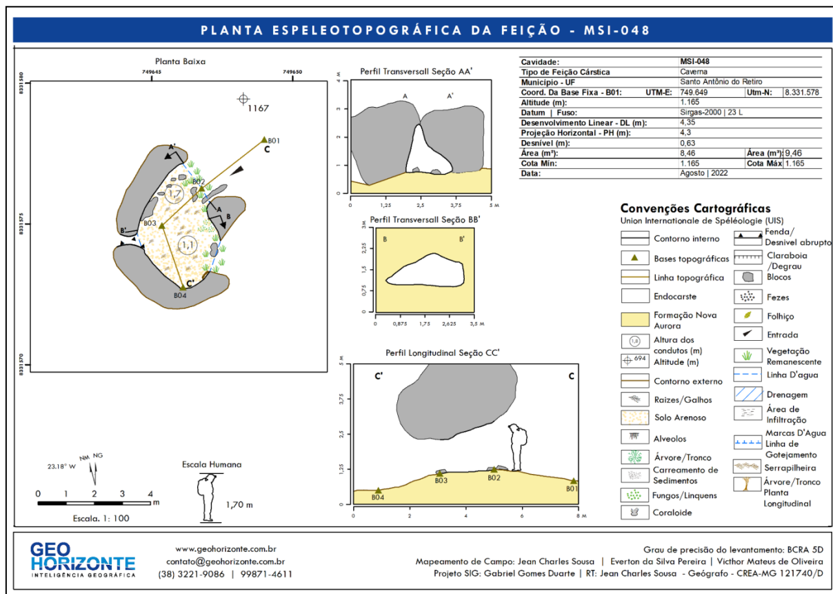
Figura 25: Planta espeleotopográfica – CNS MSI-048.
