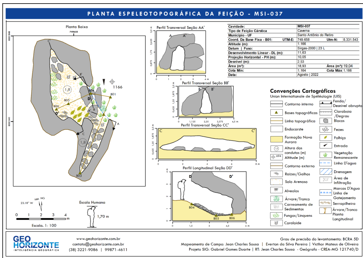
Figura 21: Planta espeleotopográfica – CNS MSI-037.
