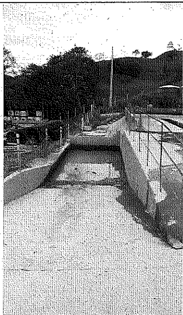
Foto 03. Rampa de decantação e Caixa SAO.
