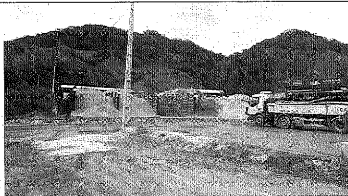
Foto 02. Baías de armazenamento de agregados.
