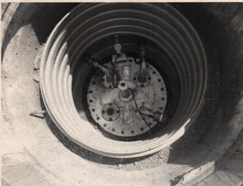
Bocas de visita com sump e fiação com instalação de monitoramento intersticial
