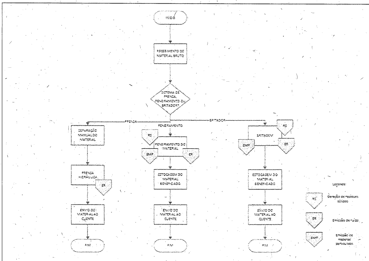
Quadro 01: Fluxograma do processo produtivo e aspectos ambientais.
