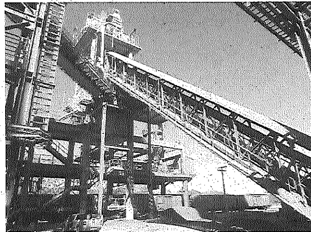
Foto 04. Correia para transporte e carregamento do clínquer excedente nos vagões.
