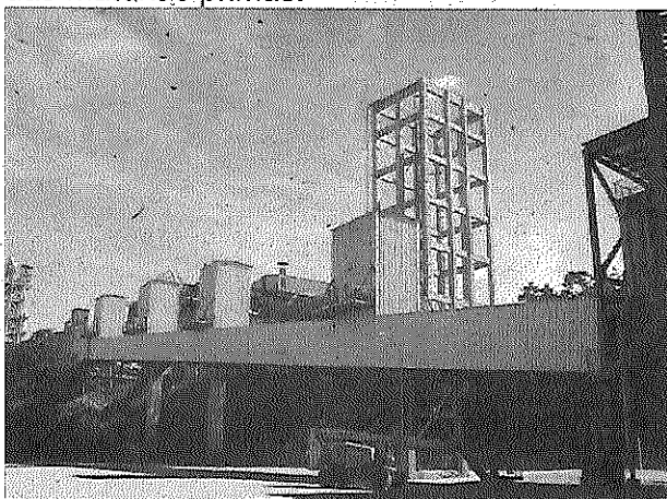
Foto 07. Sistema pneumático para transporte do cimento à área de expedição e ensacamento.
