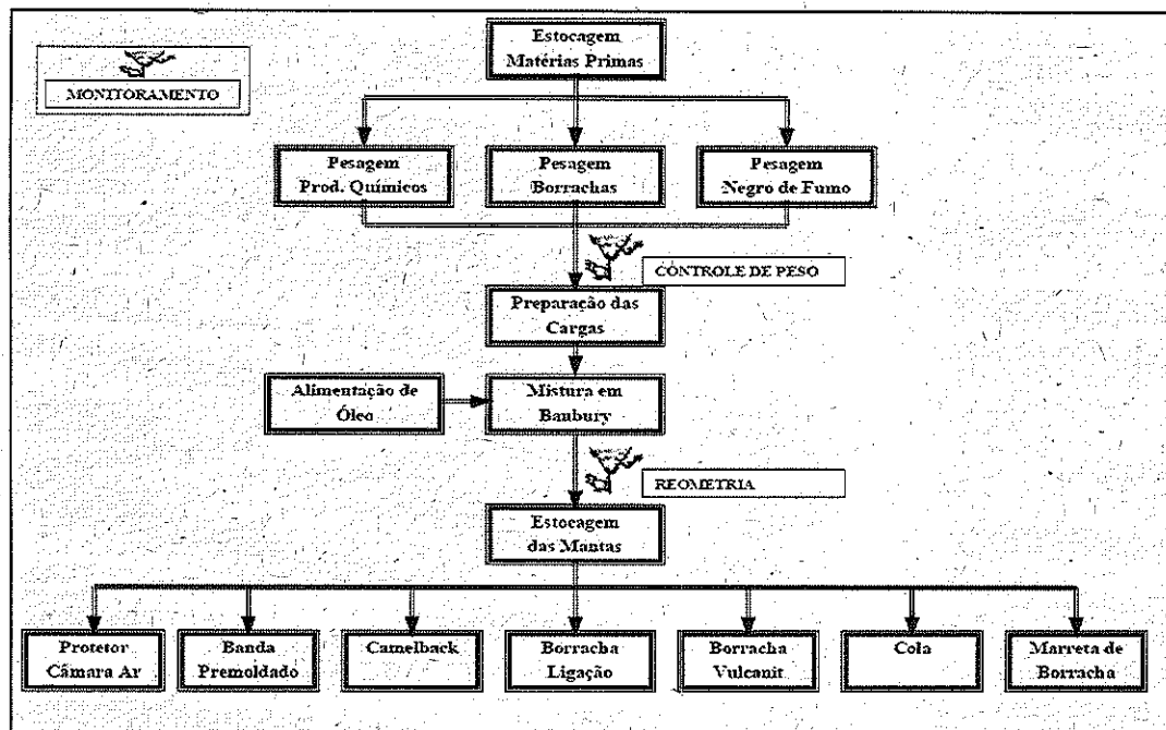
Figura 01 – Fluxograma do processo produtivo.
