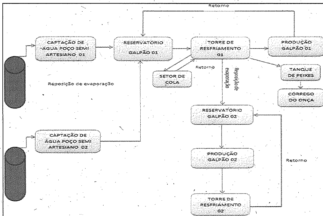
Figura 04: Fluxograma dos sistemas de recirculação de água
