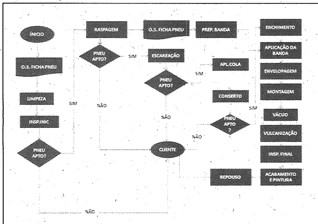
Figura 01 – Fluxograma do processo de recauchutagem de pneumáticos.
