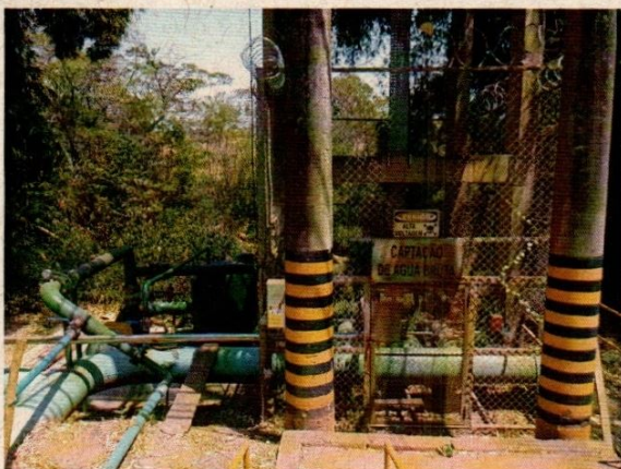
Figura 5: Captação superficial.
