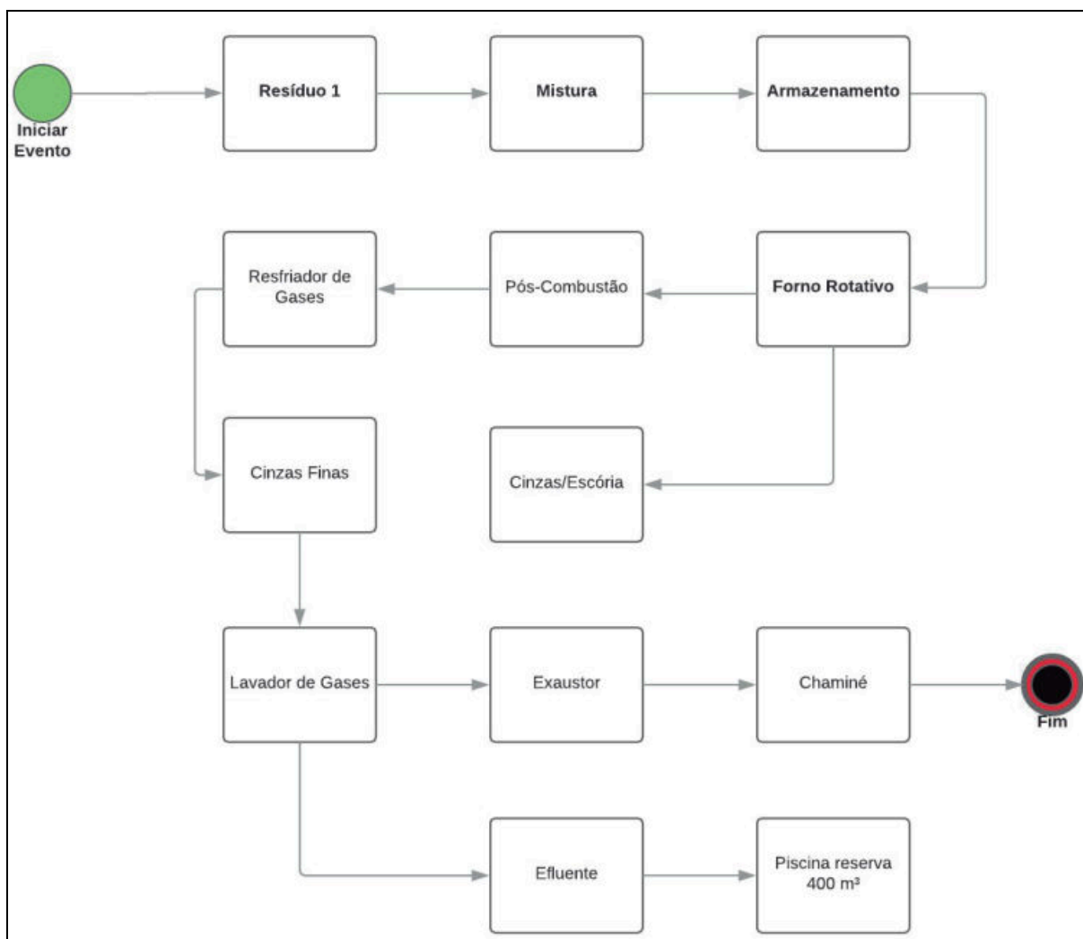
Figura 2- Esquema do fluxograma industrial. Fonte: EIA Termoambiental, 2019.
